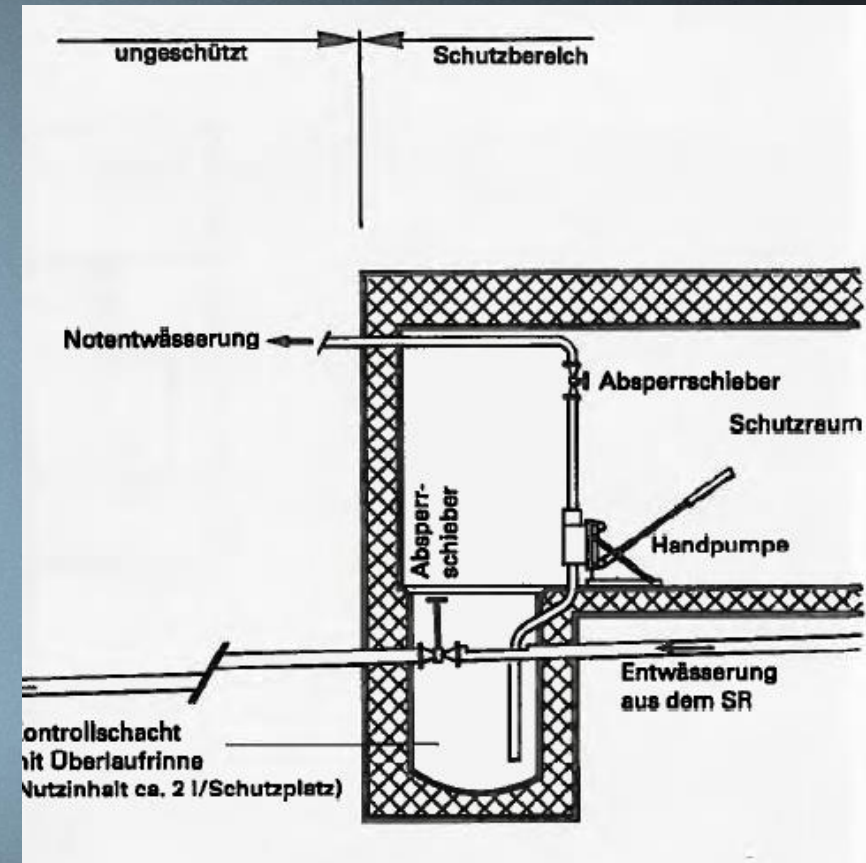
Pav. atsarginio nuotekų rezervuaro įrengimas. TWS 1982 figur 2.3-8 Technische Weisungen für Spezielle Schutzräume
