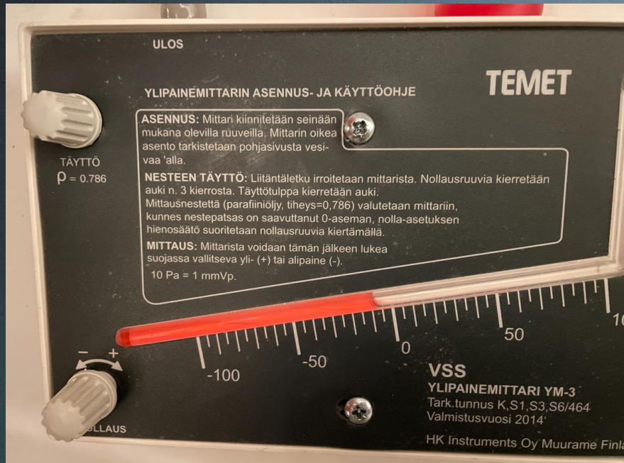
Pav. slėgių skirtumo matavimo elementas
