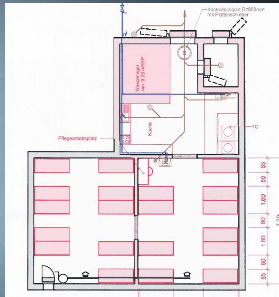
Pav. 40 vietų slėptuvė. TWS 1982 Technische Weisungen für spezielle Schutzräume
