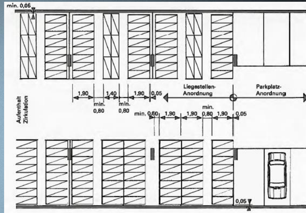
Pav. galima SPKAS gultų išdėstymo schema kai požeminės automobilių saugyklos tarpatramis sudaro 7,50 m
